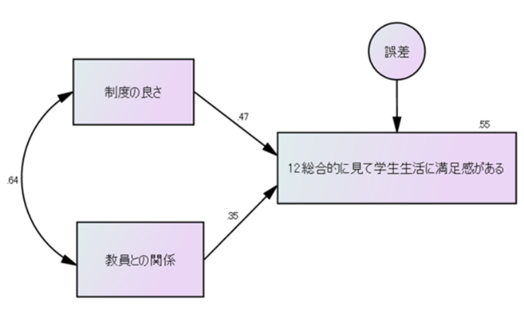
図1 重回帰分析のパス図
